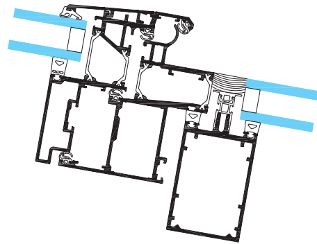
TENTAL 50 kattoikkuna
