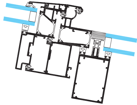
TENTAL 50 kattoikkuna
