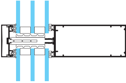
TENTAL 50 korkeaeeristetty
