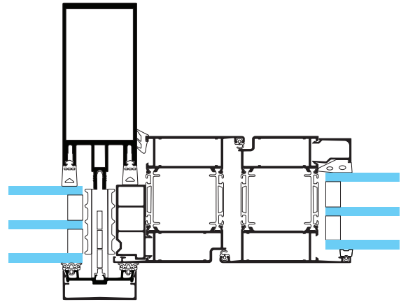
TENTAL 50 2086 oviliitoksella
