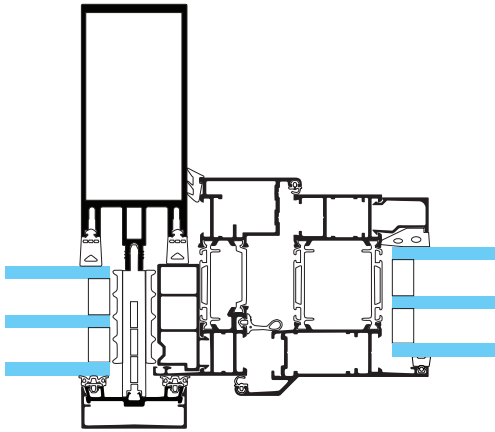
TENTAL 50 1086 ikkunaliitoksella
