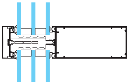
TENTAL 50 Højt isoleringsniveau
