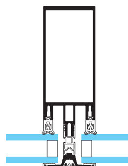
TENTAL 50 Lavt dekorprofil
