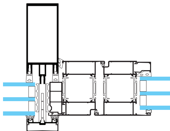
TENTAL 50 Indbygning af Sapa dør 2086
