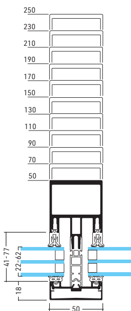
TENTAL 50 Eksempler på mulige profilstørrelser
